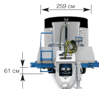
Конвейер с разгрузкой на две стороны
