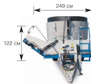
Цепной конвейер-подъемник (Разгрузка на левую сторону)
